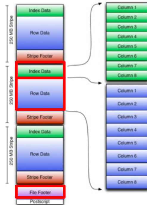
ORCのデータ構造
